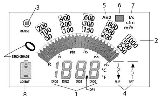
Figura 4 Pantalla LCD del LoFlo Balometer®
