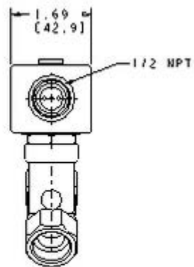
VIEW A-A
