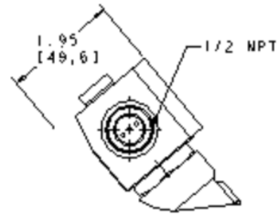
VIEW A-A
