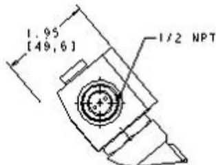
VIEW A-A
